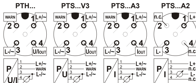
Abb. 3. A-codierter M12-Stecker
