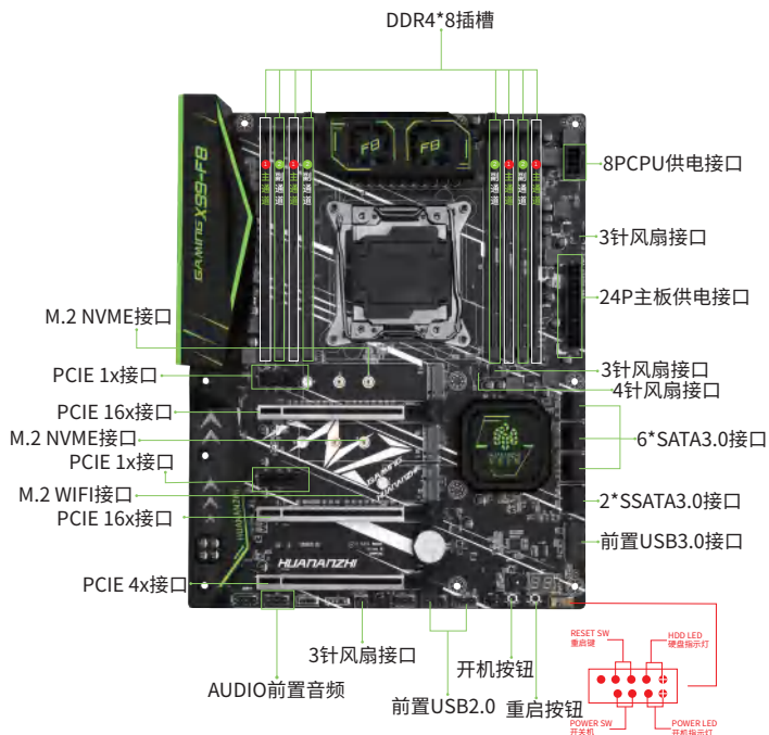
图1-1 X99-F8主板图解
