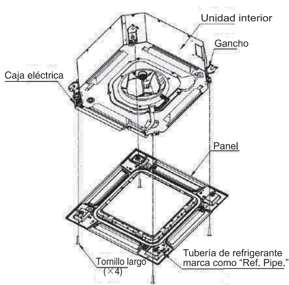
Fig. 2.3 Instalación
