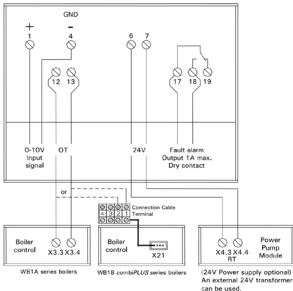
Fig. 9 Input Module wiring diagram
