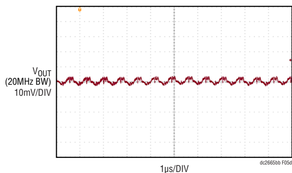
(d) 5V_{OUT} , 1.5MHz, 20MHz Bandwidth
