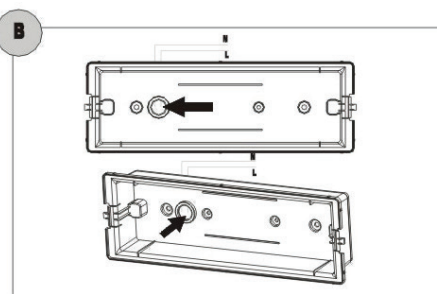
INSTALARE ASCUNSĂ
