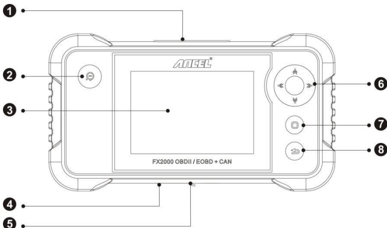
Figura 3-1 Vista frontal de FX2000
