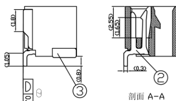
剖面 A-A
