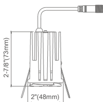
1" MODULE
