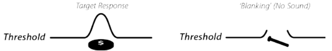
Şekil 43 – Dedektör sesleri
