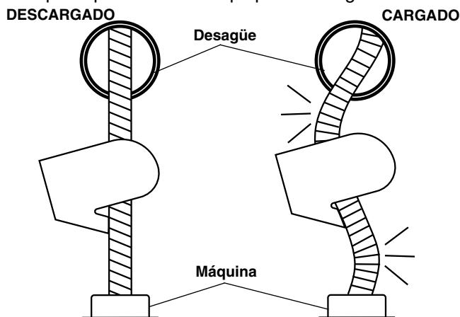
Figura 13 – Forma que adopta el cable cuando está descargado o cargado
