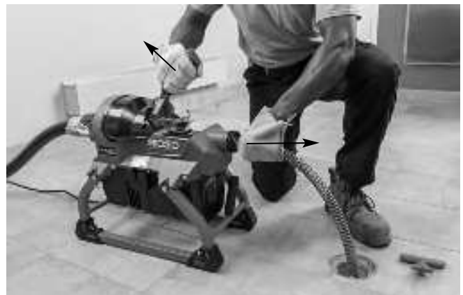
Figura 11 B – El embrague se ha soltado, el cable no está girando y el operario está jalando el cable para extraerlo de la máquina
