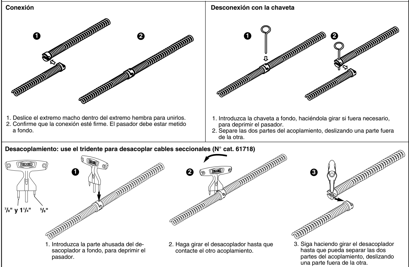
Figura 8 – Acoplamiento y desacoplamiento
