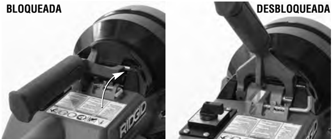
Figura 4 – Liberación de la manilla del embrague
