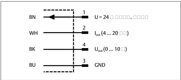
Рис. 4: Жилы кабеля
