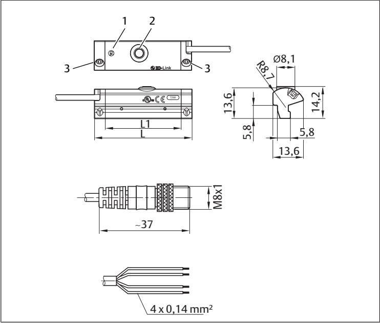
Рис. 1: Размеры
