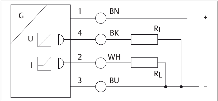
Рис. 3: Разводка контактов
