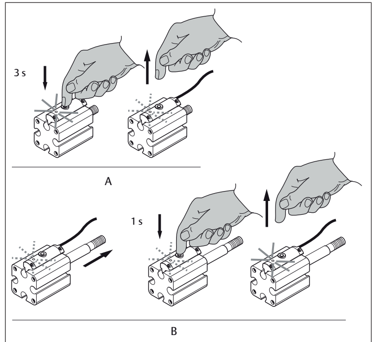
Fig. 5: Aprendizaje del punto cero (A) / aprendizaje del punto final (B)
