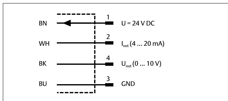
Bild 4: Kabeltrådar
