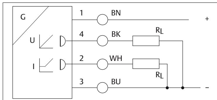
Bild 3: Stiftstilldelning
