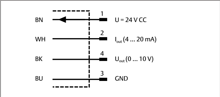
Fig. 4: Fils de câbles
