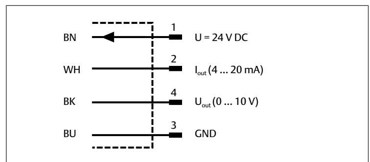
Abb. 4: Kabeladern
