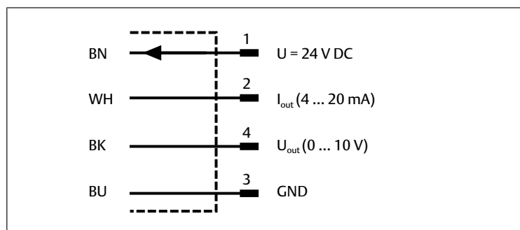
Fig. 4: Fili del cavo
