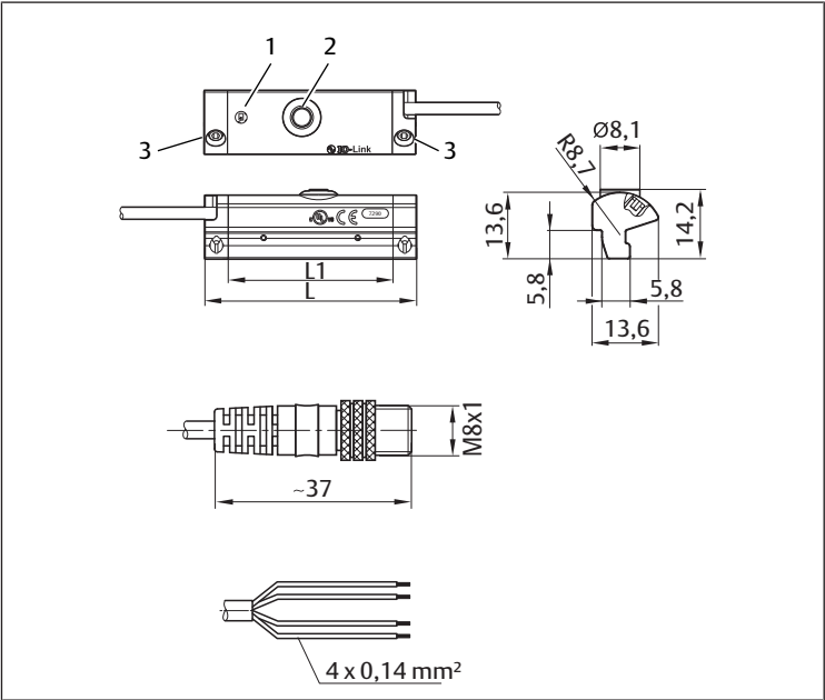
Bild 1: Mått
