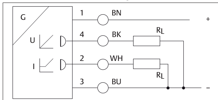
Fig. 3: Occupazione connettori
