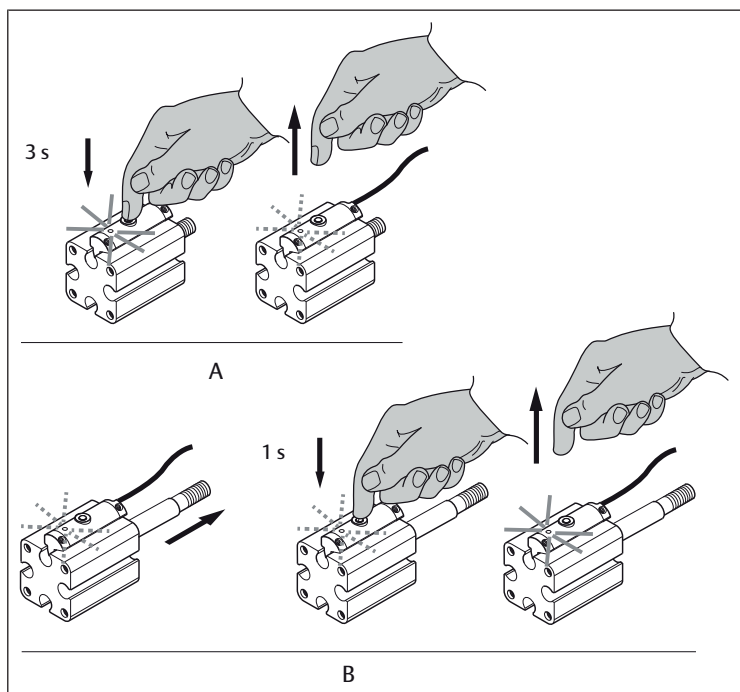
Fig. 5: Apprentissage du point zéro (A) / Apprentissage du point final (B)
