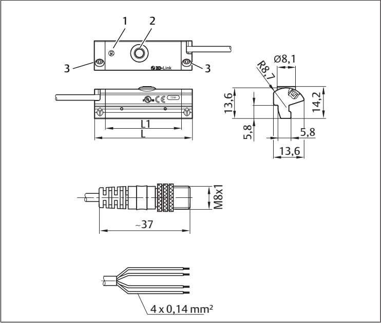
Fig. 1: Dimensions
