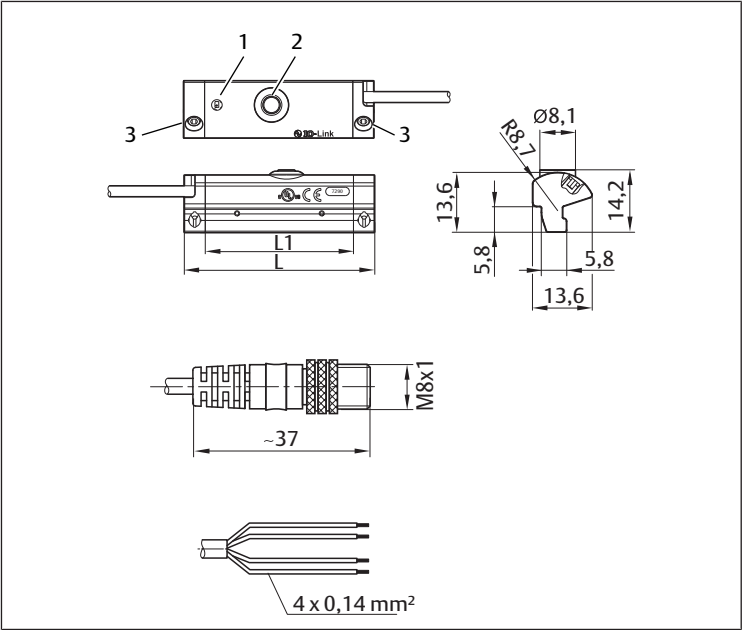
Fig. 1: Dimensioni
