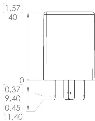
Seitenansicht
