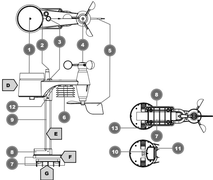
Abb. 2: Alle Teile des Multisensors
