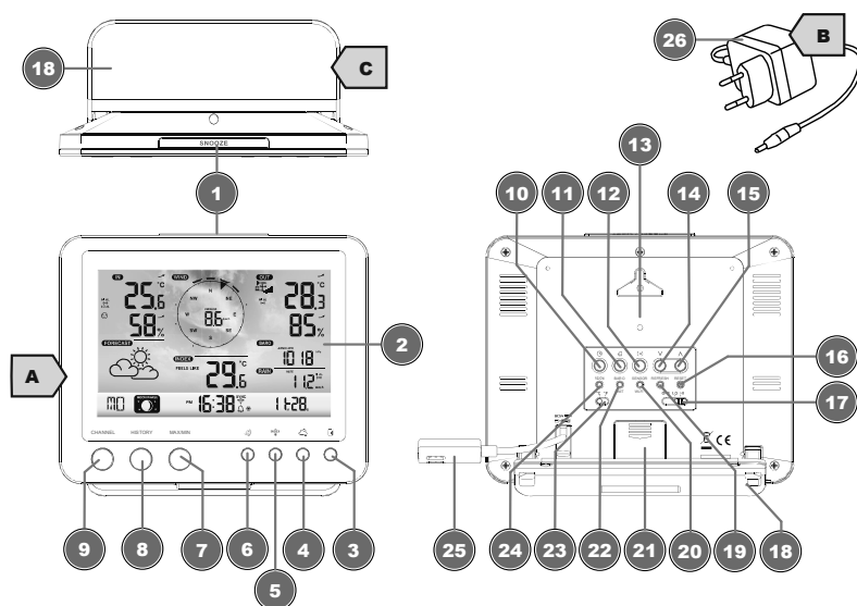
Abb. 1: Alle Teile der Basisstation
