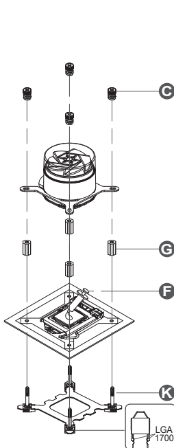
Intel LGA 1700
