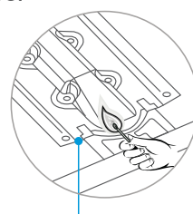
Quemador de la cavidad inferior
