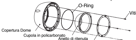
Figura : Assemblaggio cupola del dome
