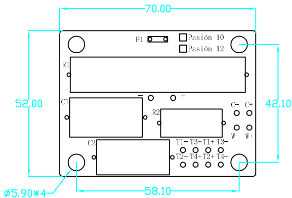
PCB-零件面 /components side
