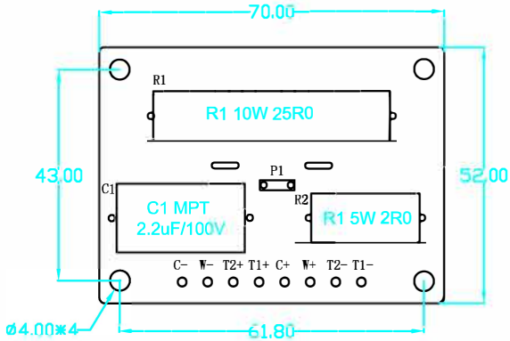
PCB-零件面 /components surface
