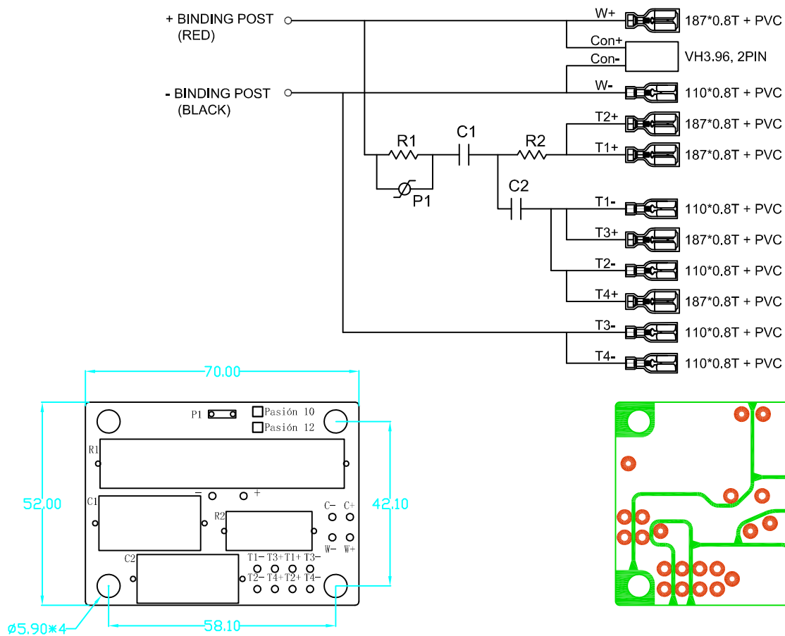
PCB-零件面 /components surface
