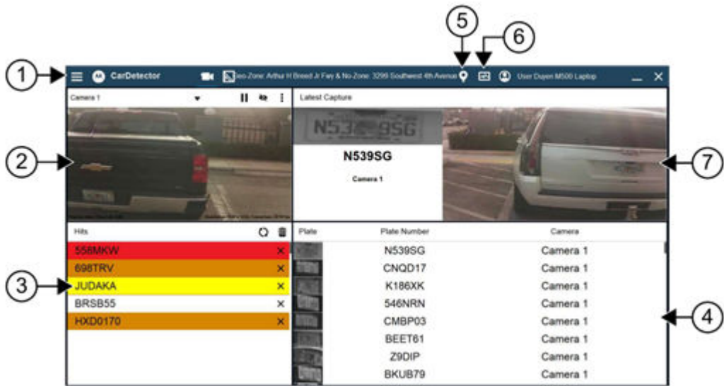
Figura 5: Descripción general de la interfaz principal de CarDetector
