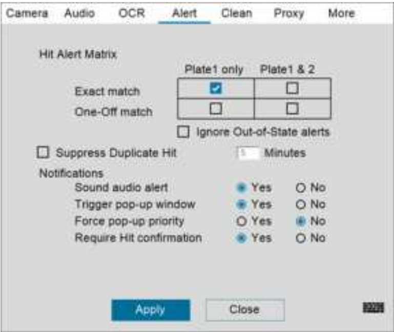
Mesa 9: Descripción del menú Configuración de alertas
