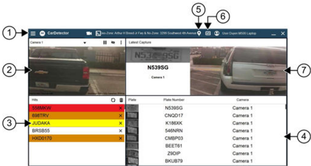
Figura 5: Visão geral da interface principal do CarDetector
