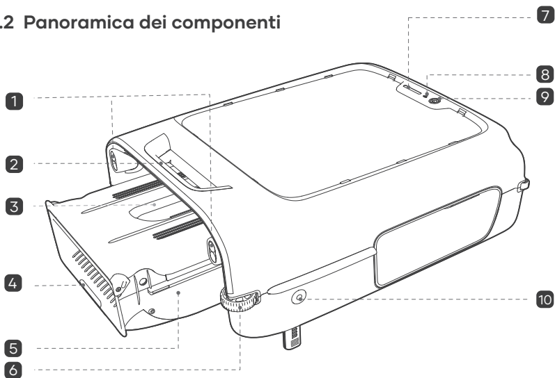
Skimmer (vista laterale)
