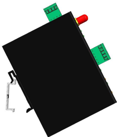
DIN Rail Assemblying
