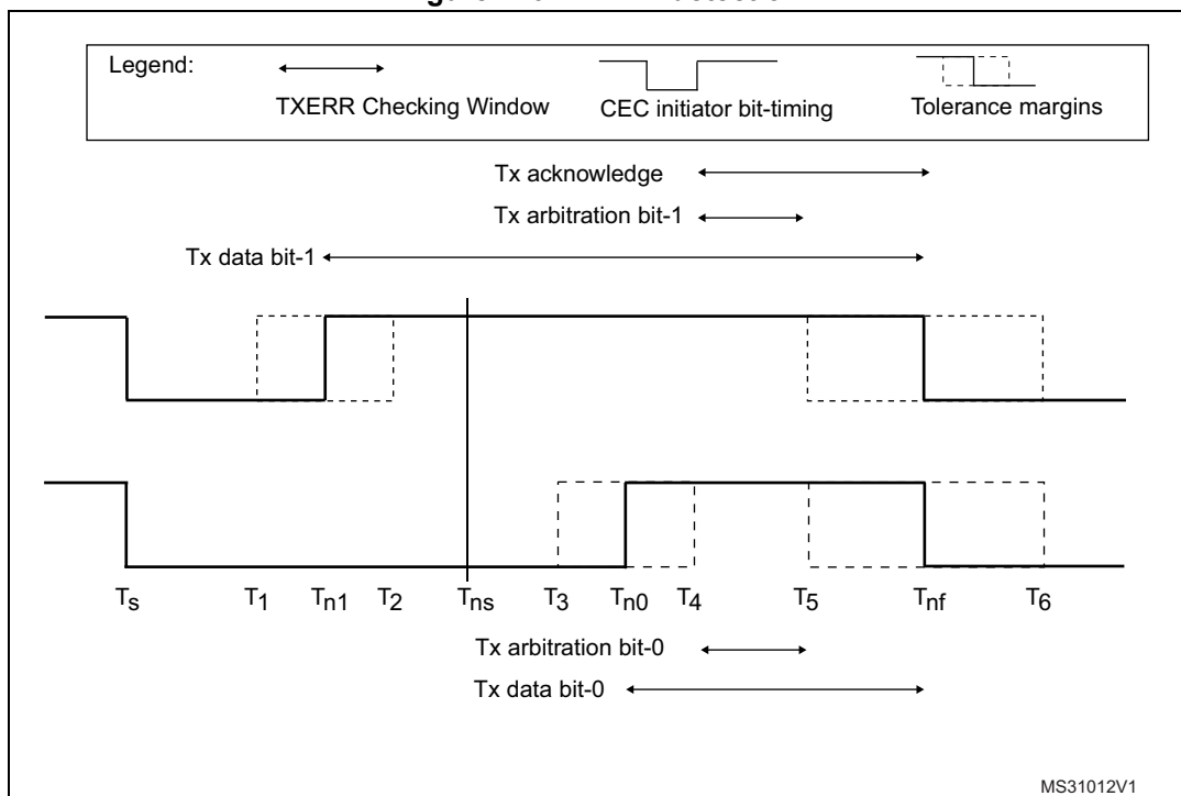
Figure 440. TXERR detection
