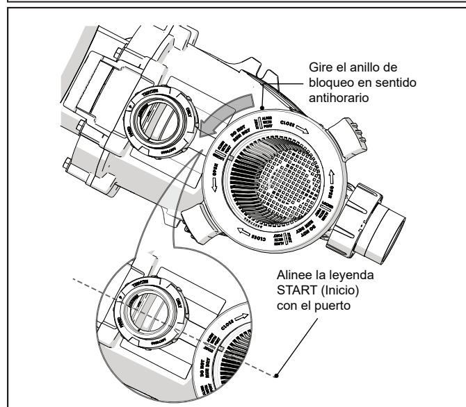
Figura 17. Desconectar el anillo de bloqueo
