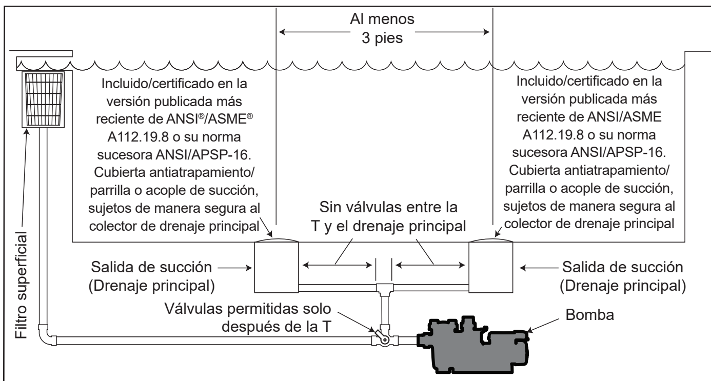
Figura 4. Cantidad de salidas de succión por bomba
