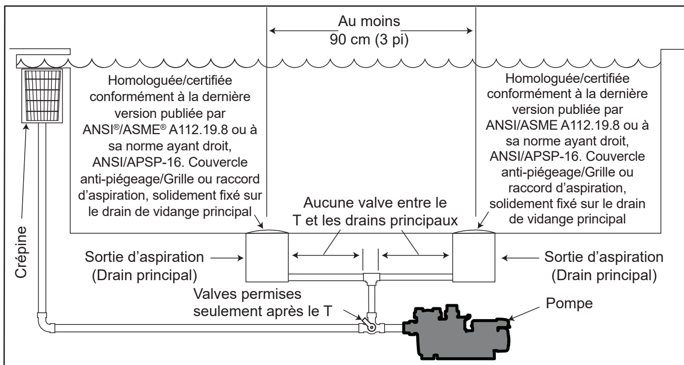
Figure 4. Nombre de prises d'aspiration par pompe
