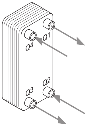
Skraplacz
