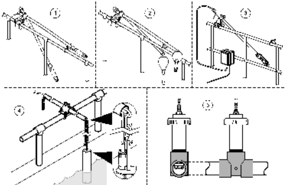
그림 5 설치 옵션
