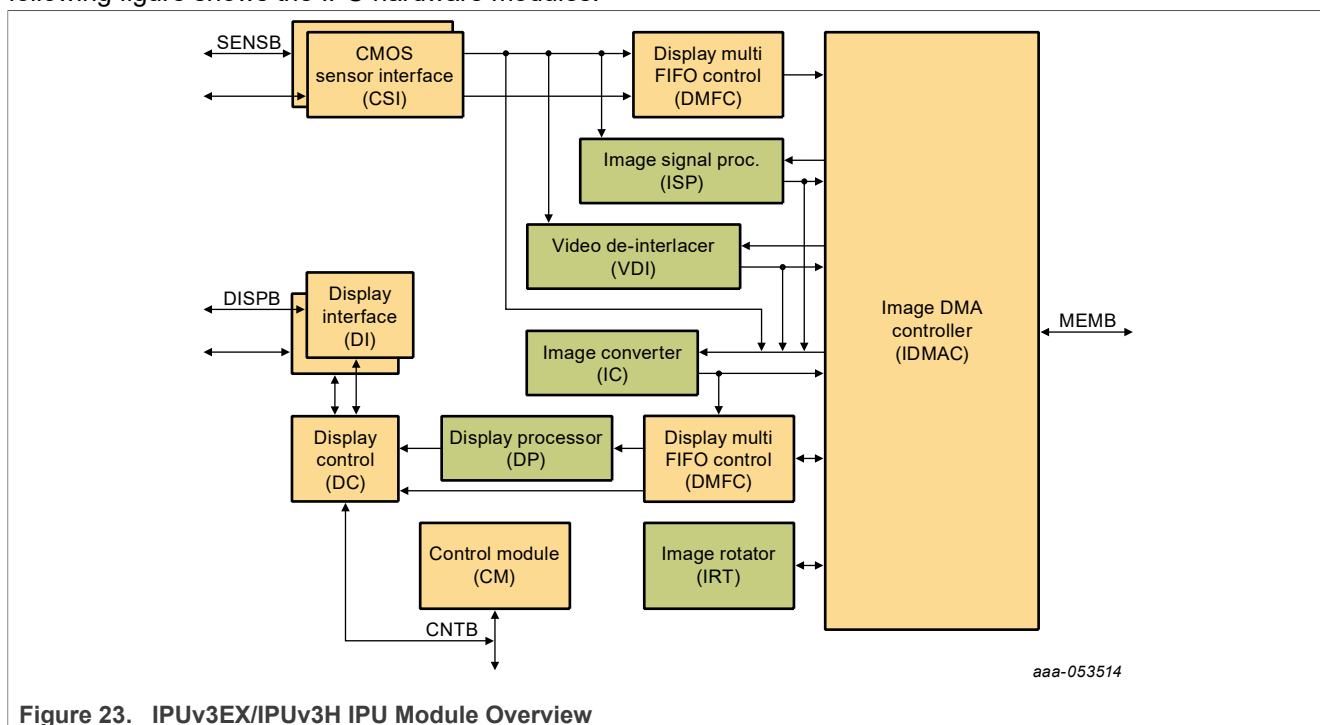
Figure 23. IPUv3EX/IPUv3H IPU Module Overview
