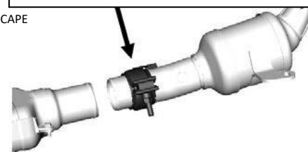
SUJETADOR DE CONECTOR DE CONVERTIDOR CATALÍTICO DEL LADO IZQUIERDO
