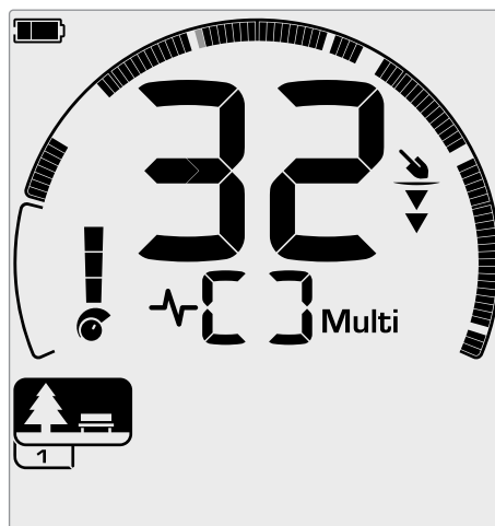
Ejemplo de detección de un objetivo no ferroso aceptado con un ID de objetivo de 32. El segmento 32 de la escala de discriminación parpadeará.
