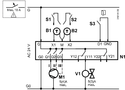
1-speed or 3-speed fan
