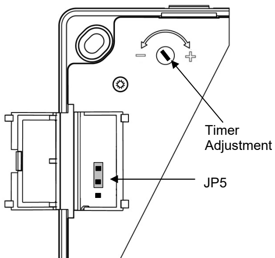
Fig.5: VASF100BO , VASF100TO
