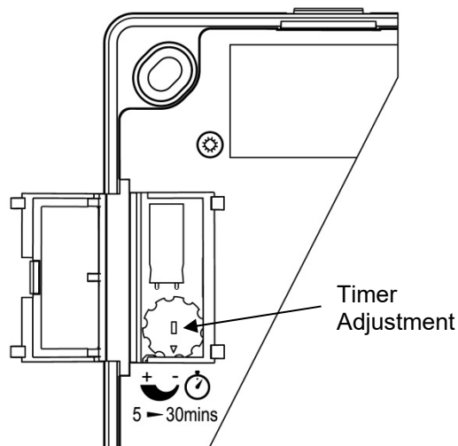
Fig. 4: PIR TIMER
