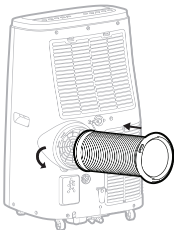
Tubo de escape: Diámetro: 5,9" (15 cm) Longitud: 10,23" a 47" (26 cm a 120 cm)
