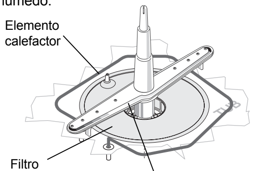
Conjunto del brazo rociador/torre
