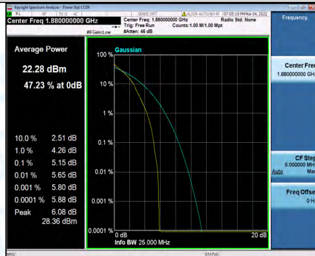
Band2-20MHz-QPSK-18900-100RB#0
