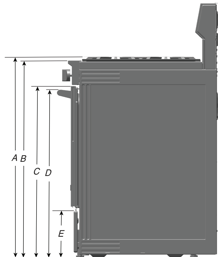
VUE LATÉRALE
