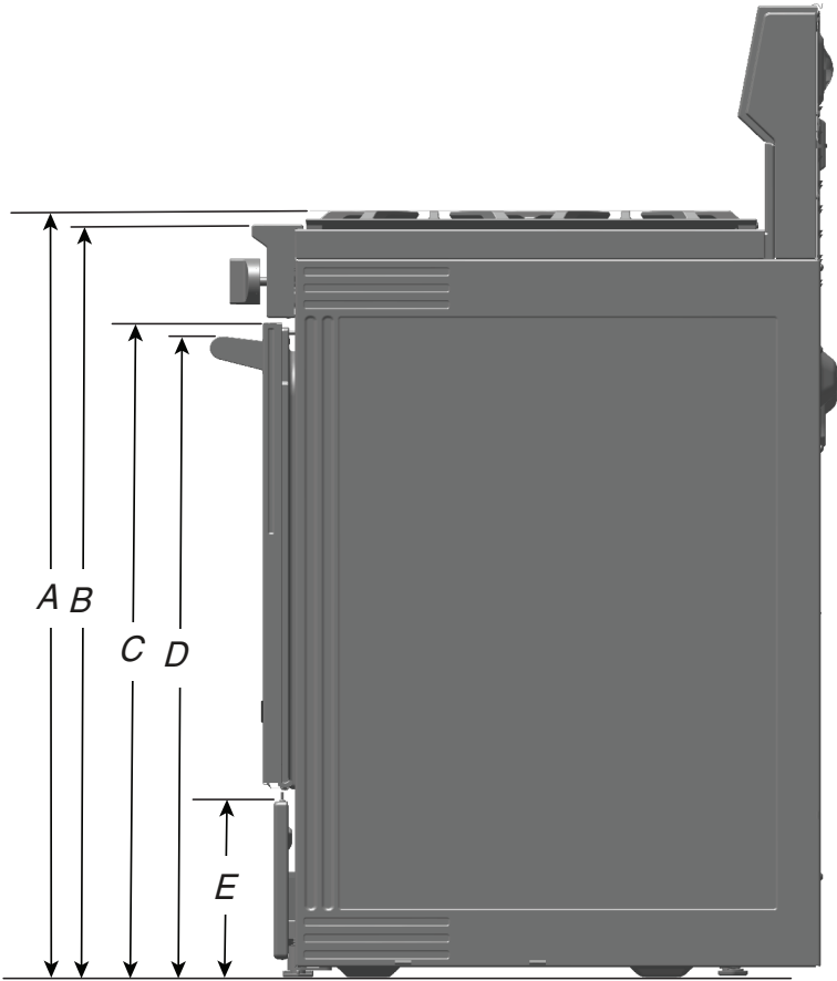
VISTA LATERAL
