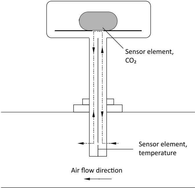
Fig. 1 L'écoulement d'air peut être dirigé de droite à gauche (comme dans l'exemple ci-dessus) ou de gauche à droite.
