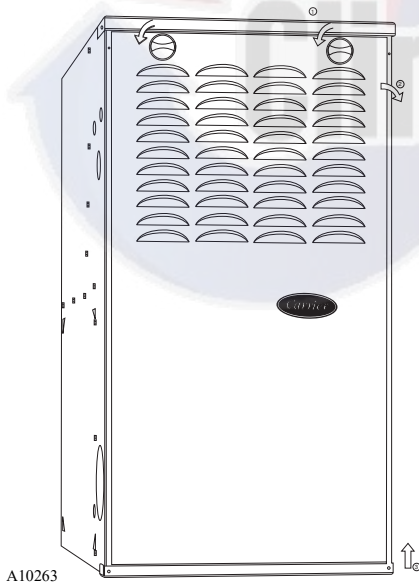
Fig. 7 – Remove Furnace Door
