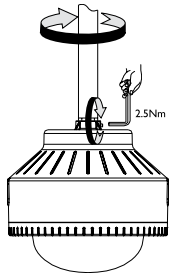
Монтаж на трубе
