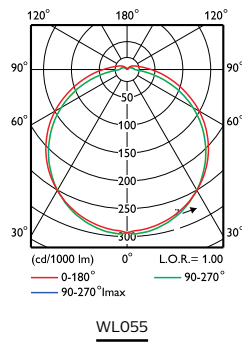
Фотометрическая кривая в полярных координатах
