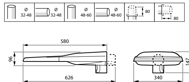
UNI LUMISTREET GEN2_MEDIUM 62
