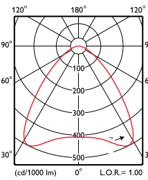
BY718P LED100 WB
