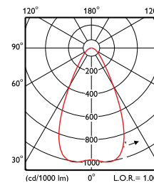
BY718P LED100-LED150 NB
