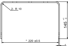
Монтажная скоба BY200Z MB
