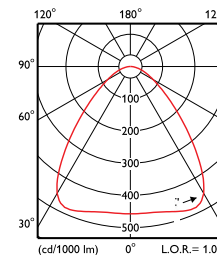
BY718P LED150-LED200 WB
