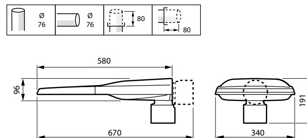
UNI LUMISTREET GEN2_MEDIUM 76
