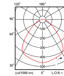
BY718P LED250-LED300 WB
