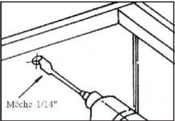
Schéma 8: Perceur un trou d'accès pour la ligne électrique
