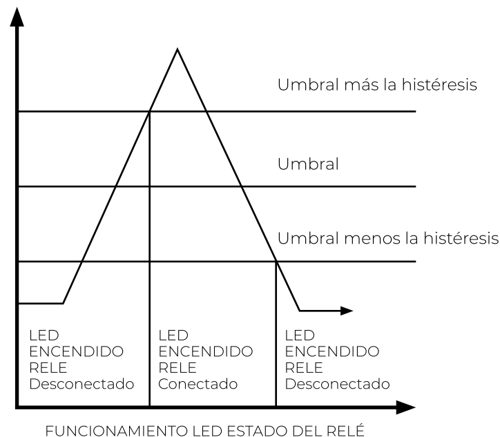
FUNCIONAMIENTO LED ESTADO DEL RELÉ
