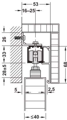
Wall mounting with mounting bracket and fixing clip for wooden panel การติดตั้งบนผนังด้วยเฟลทติดผนังและฝาปิด แบบคลิปสำหรับบานไม้
