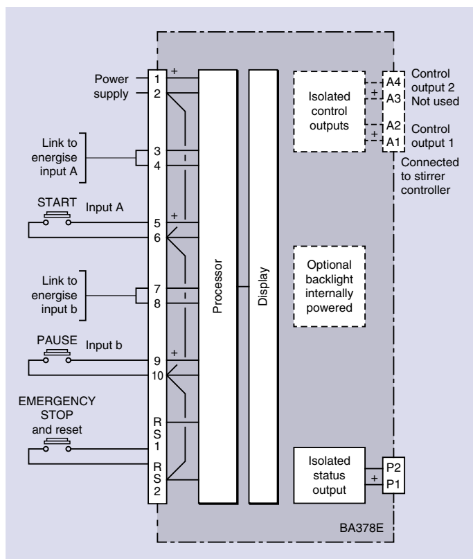
Fig 11 Timer wiring
