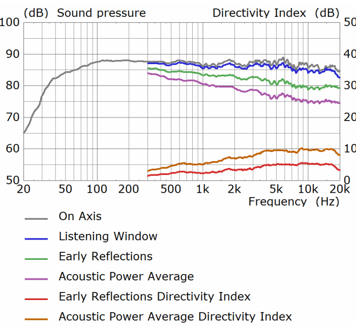
R5 Meta Spinorama
