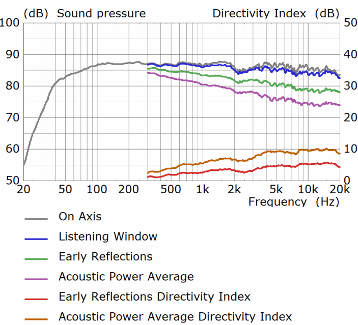
R3 Meta Spinorama
