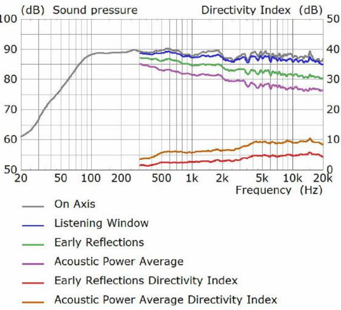
R6 Meta Spinorama
