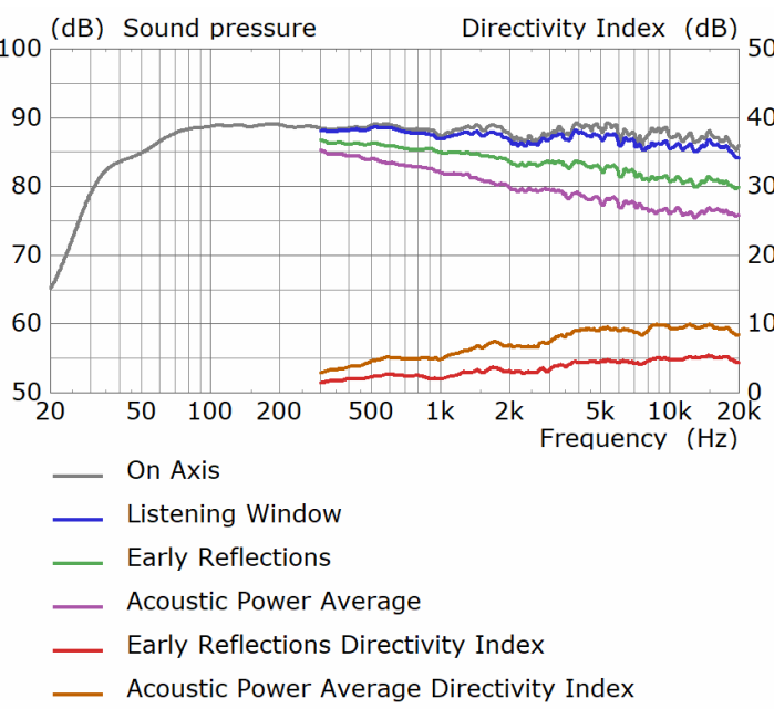
R7 Meta Spinorama
