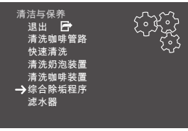
图5： 调用“除垢”程序
