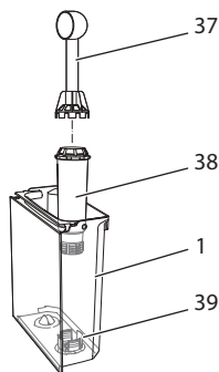
Joon. 18: Veefiltriga paigaldamine ja mahavõtmine
