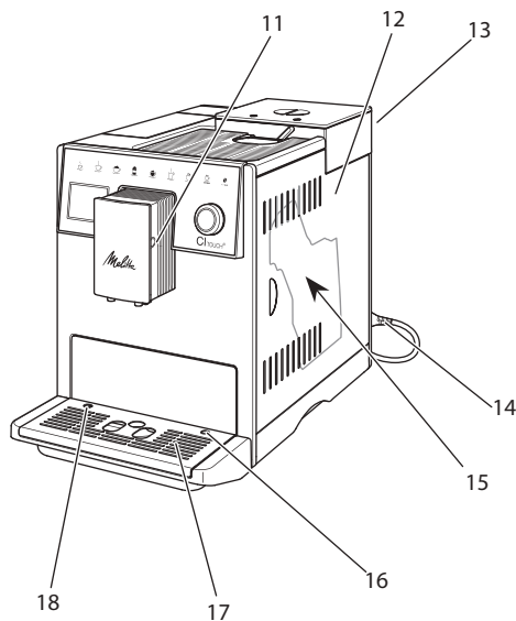
Bild 2: Kaffemaskinens framsida från höger
