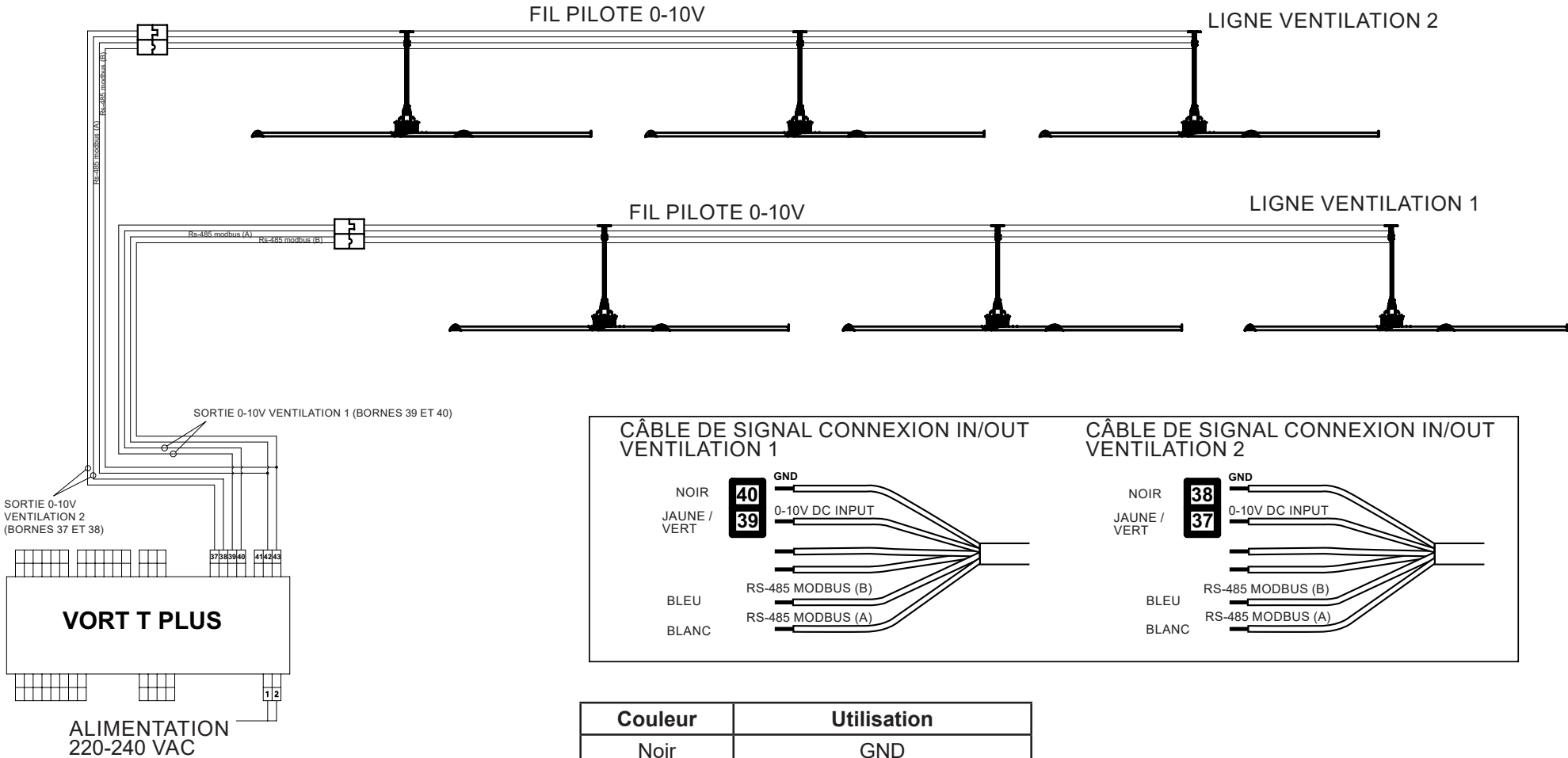
SCHEMA CONNEXIONS AVEC CENTRALE "VORT T PLUS" COD. 20.152
