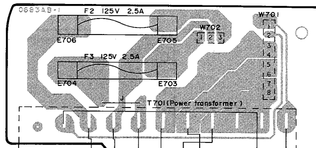
O FUSE P.C.B.
