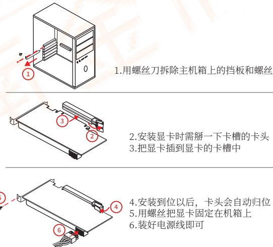
图2-10 显卡安装
