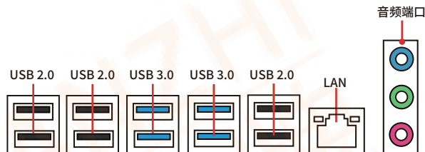
图1-2 整体后置I/O面板展示
