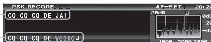
Schermata AF-FFT (pag. 41) (spettro o a caduta)
