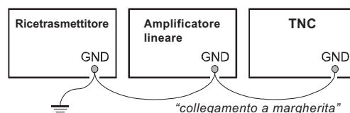
CONNESSIONE DI MASSA IMPROPRIA
