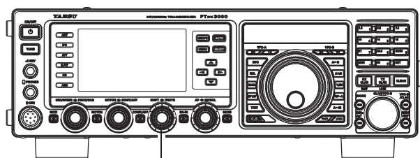
Manopola [WIDTH]
