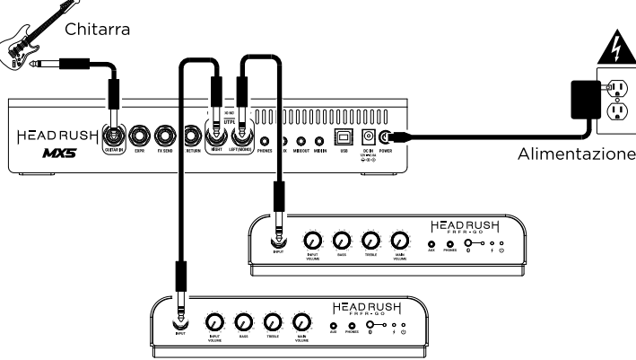
Esempio B: Due FRFR-GO (Stereo)
