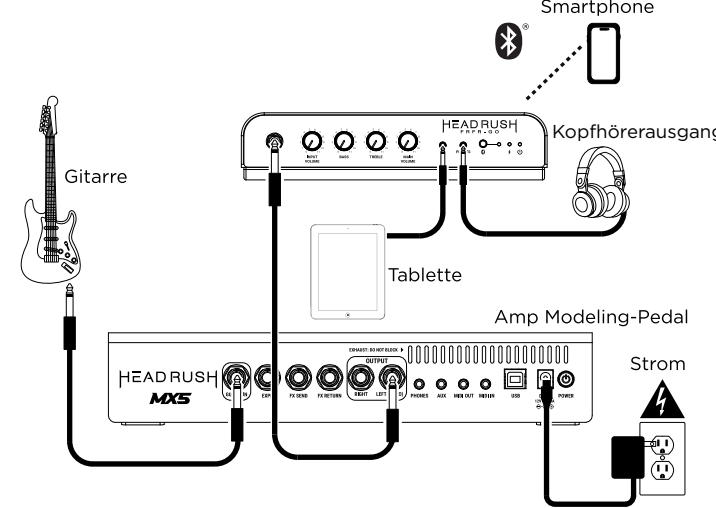
Beispiel A: Ein FRFR-GO (Mono)
