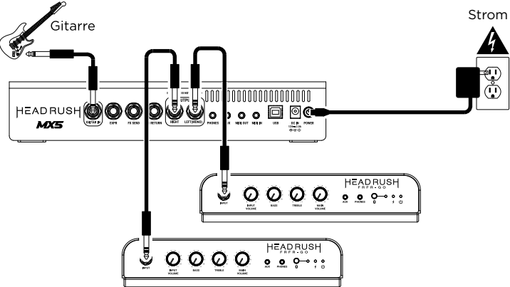
Beispiel B: Zwei FRFR-GO (stereo)
