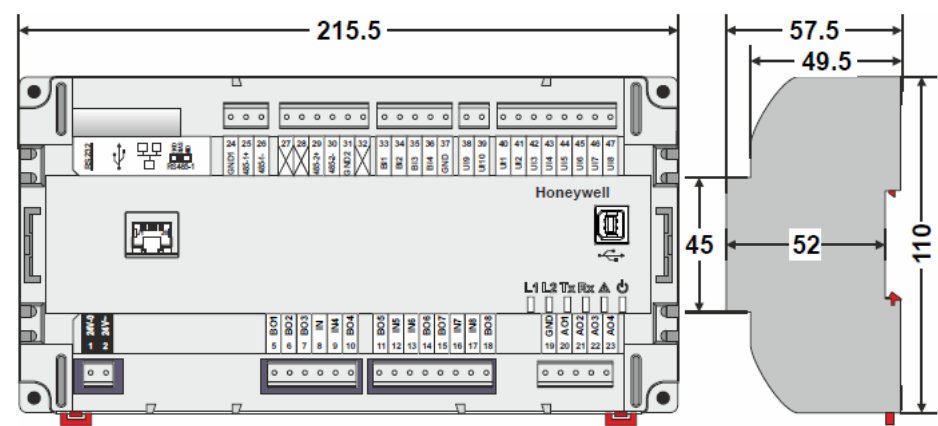
带 RJ45 接口的 MVCweb 控制器
