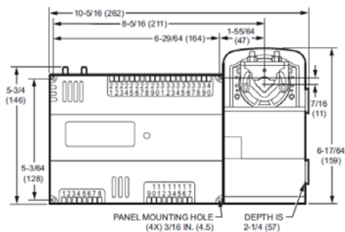
图 1: PVL6436AS 的墙面安装及尺寸 (mm)
