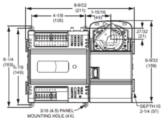
图 3: PUL1012S, PUL4024S 和 PVL4024NS
