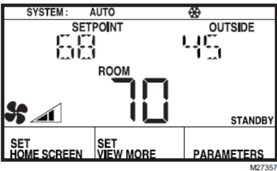
图 7 工程模式下的系统状态显示、温度设定点、室外温度和室内温度（突出显示）
