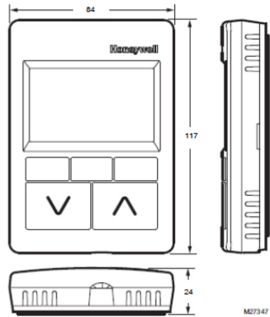
图 2 液晶显示温控单元尺寸 (mm)
