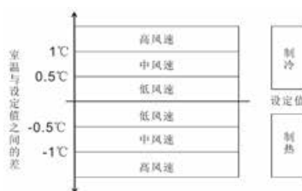
图1. 自动风速控制算法
