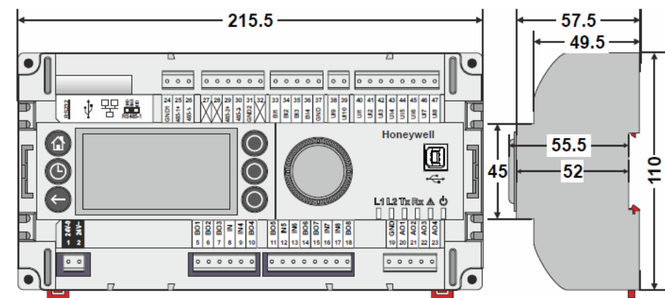
带 HMI 的 MVCweb 控制器
