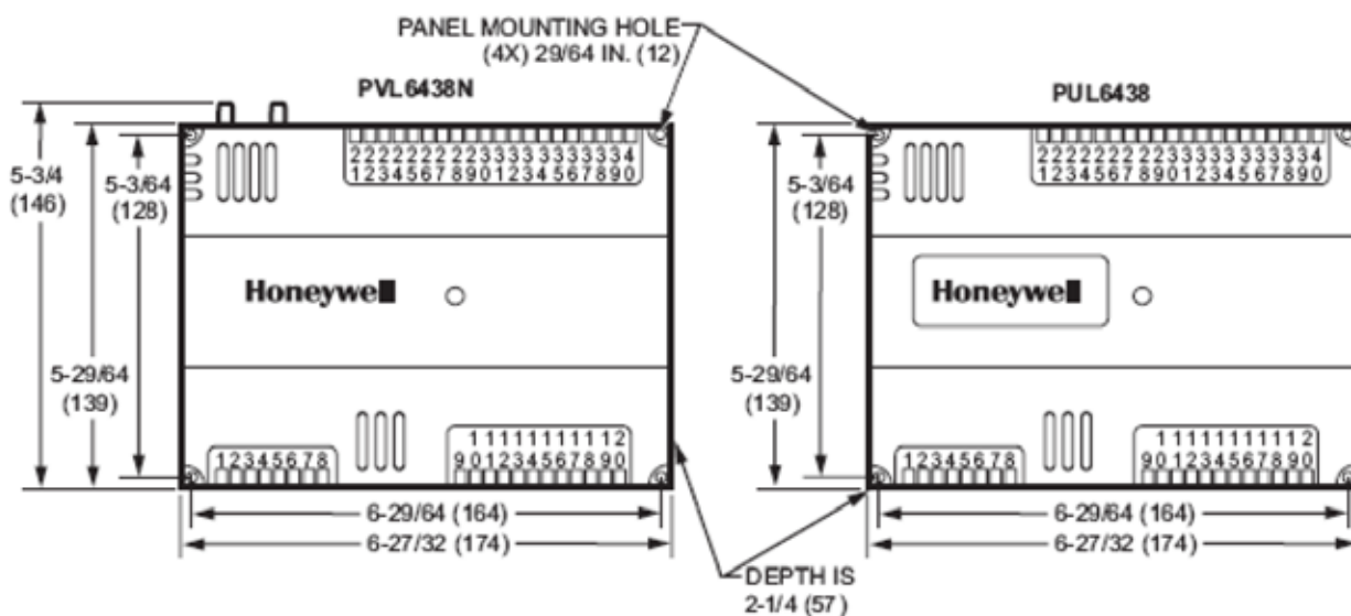
图 4: PVL6438NS 和 PUL6438S 的墙面安装及尺寸 (mm)
